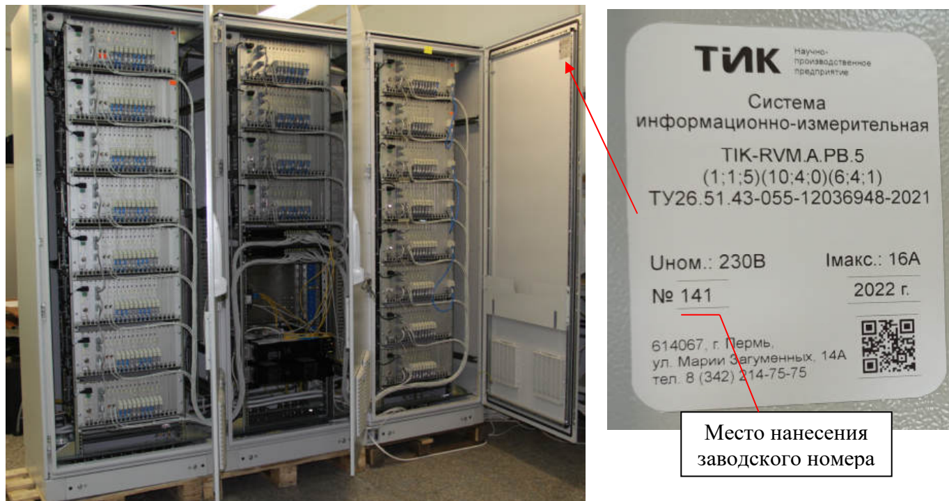
Рисунок 6 – Внешний вид шкафа систем ТИК-RVM в распределенном исполнении, место нанесения заводского номера, модификации и измерительного исполнения
